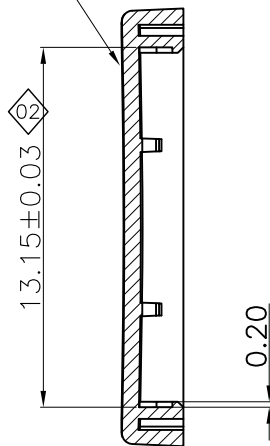
剖面 B-B
