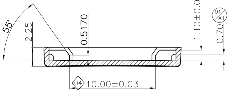
剖面 A-A
